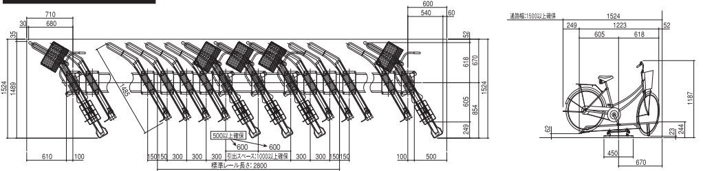
CCG II-L30型 基本寸法図
