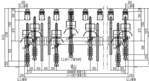
CCGII下段平面図
