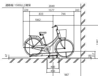
L側面図
