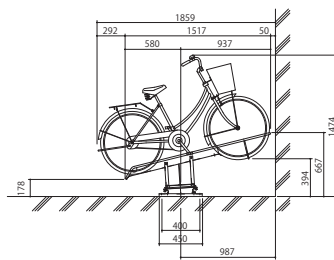
H側面図
