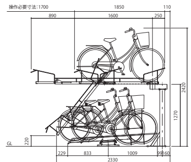
L側面図
