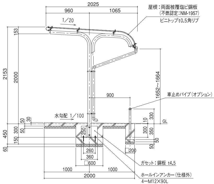
矩計図
