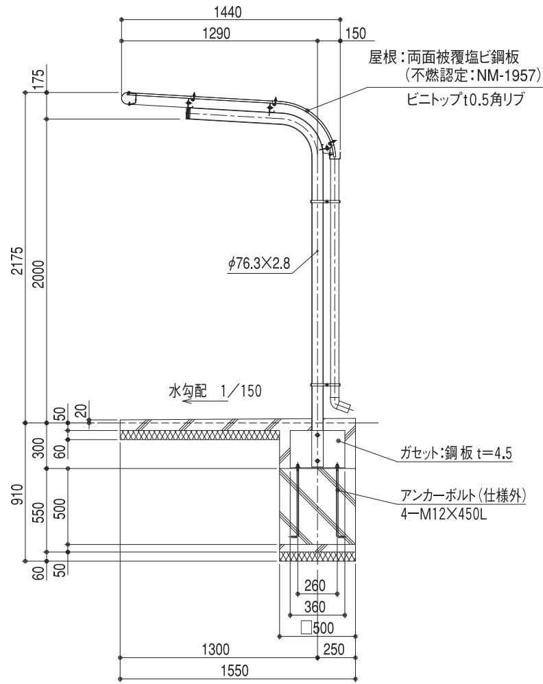
矩計図
