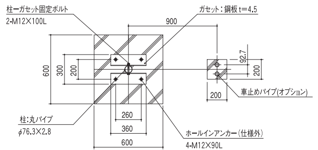
基礎部平面図
