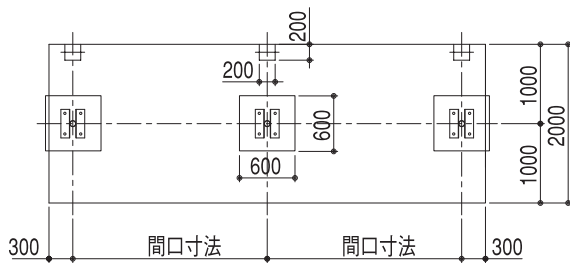
基礎伏せ図
