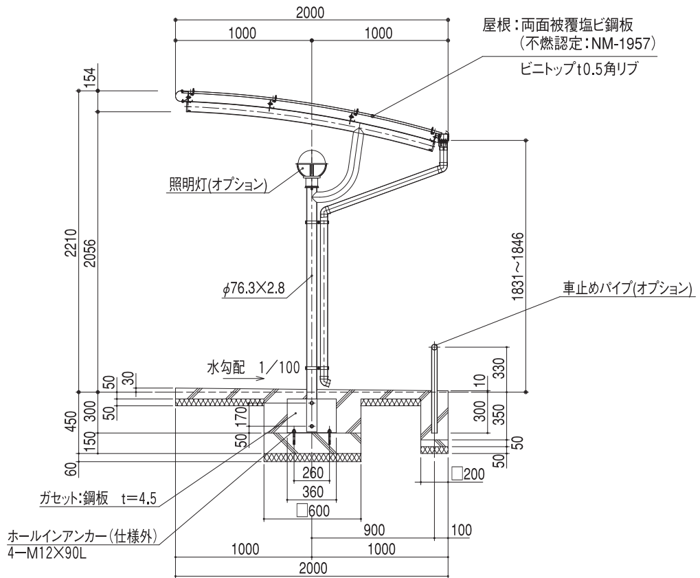
矩計図
