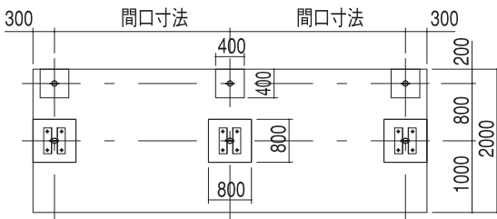
基礎伏せ図
