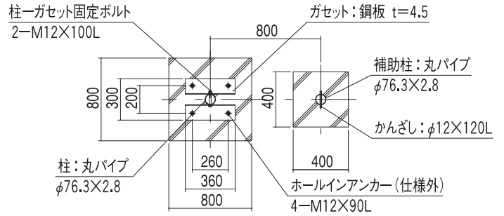
基礎部平面図
