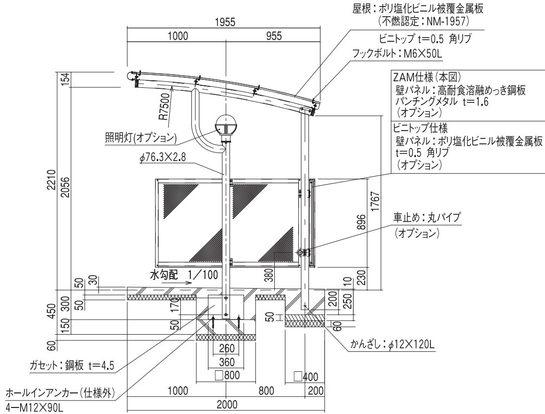
矩計図
