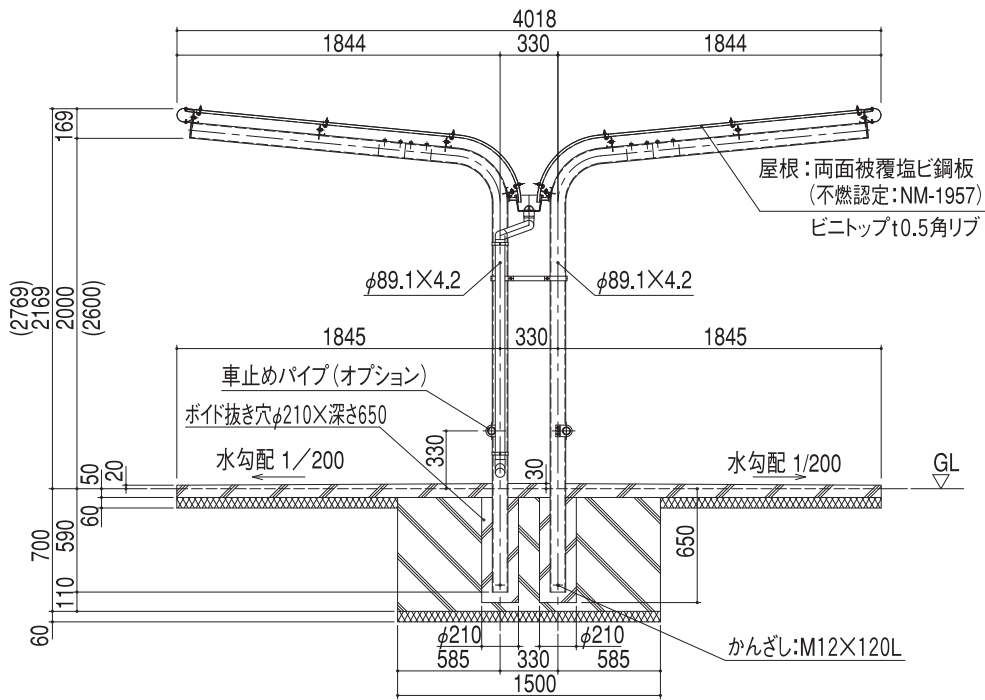
矩計図
