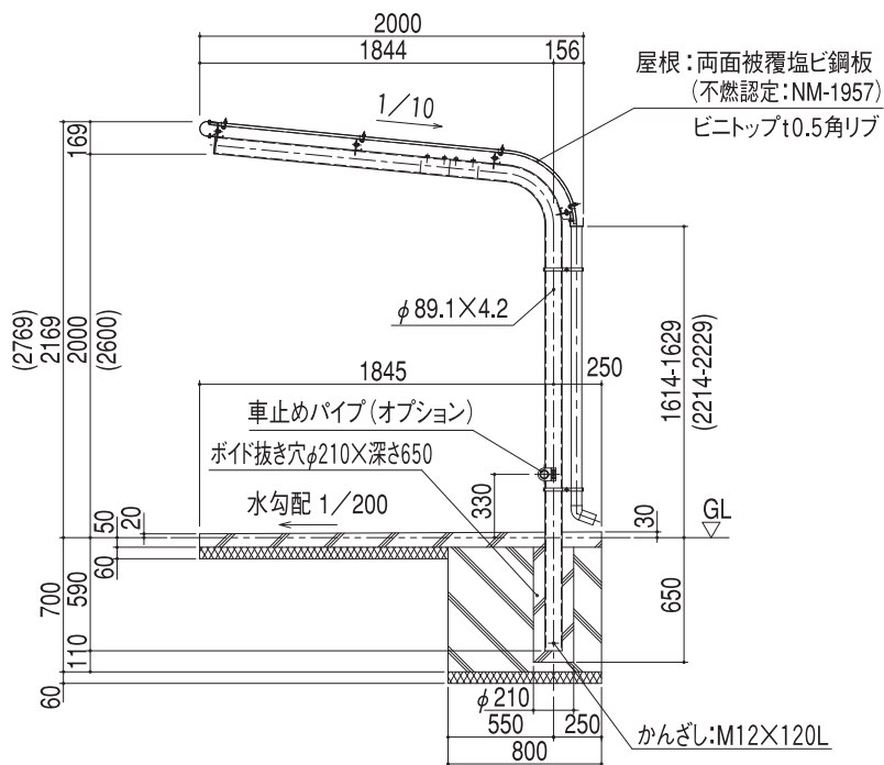
矩計図
