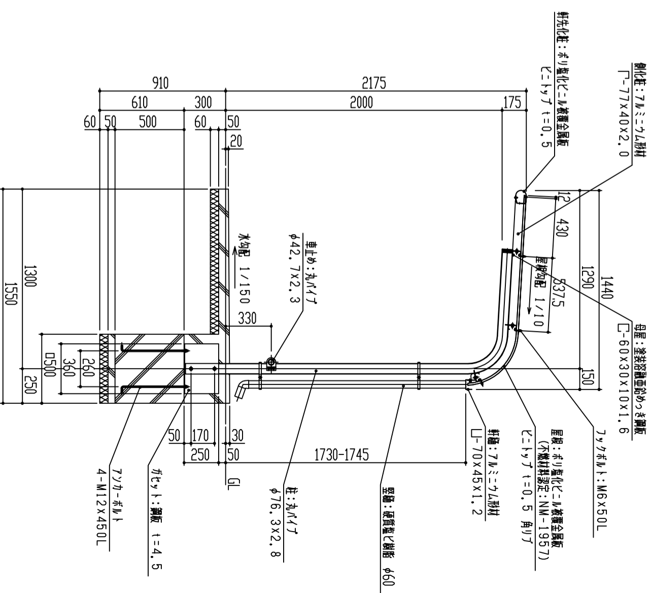
矩計図 S = 1 / 2.0
