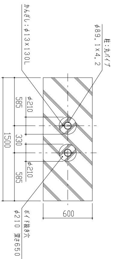
基礎部詳細図 S = 1 / 20
